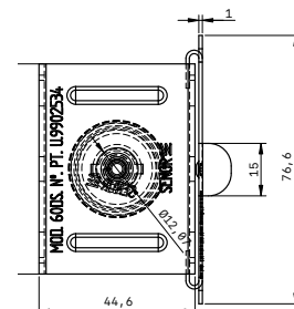
VISTA PLANTA
